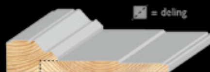
Kop- en Deellijst 28 x 140 mm
